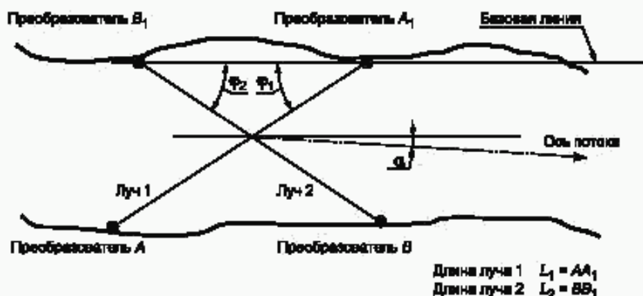
Рисунок 1 — Схема расположения преобразователей с пересекающимися лучами
