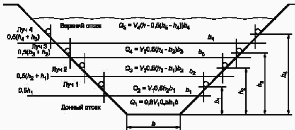
Рисунок 3 — Пример расчета расхода методом послойных сечений
